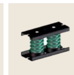
Soportes antivibratorios tipo muelle Samurai L condensación por aire Ref.: CHL-AVS-06 (tamaños 60-70) CHL-AVS-07 (tamaños 80-90) CHL-AVS-07 (tamaños 120-140)
